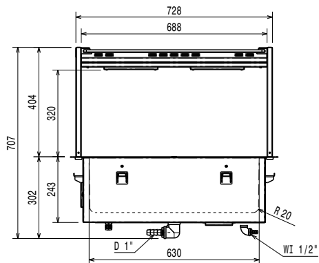
Bočna/o
